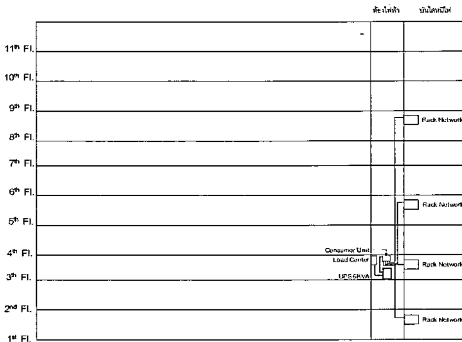
แบบติดตั้งเครื่องสำรองไฟฟ้า (UPS) อาคาร 7
