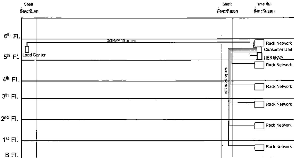
แบบติดตั้งเครื่องสำรองไฟฟ้า (UPS) อาคาร 8
